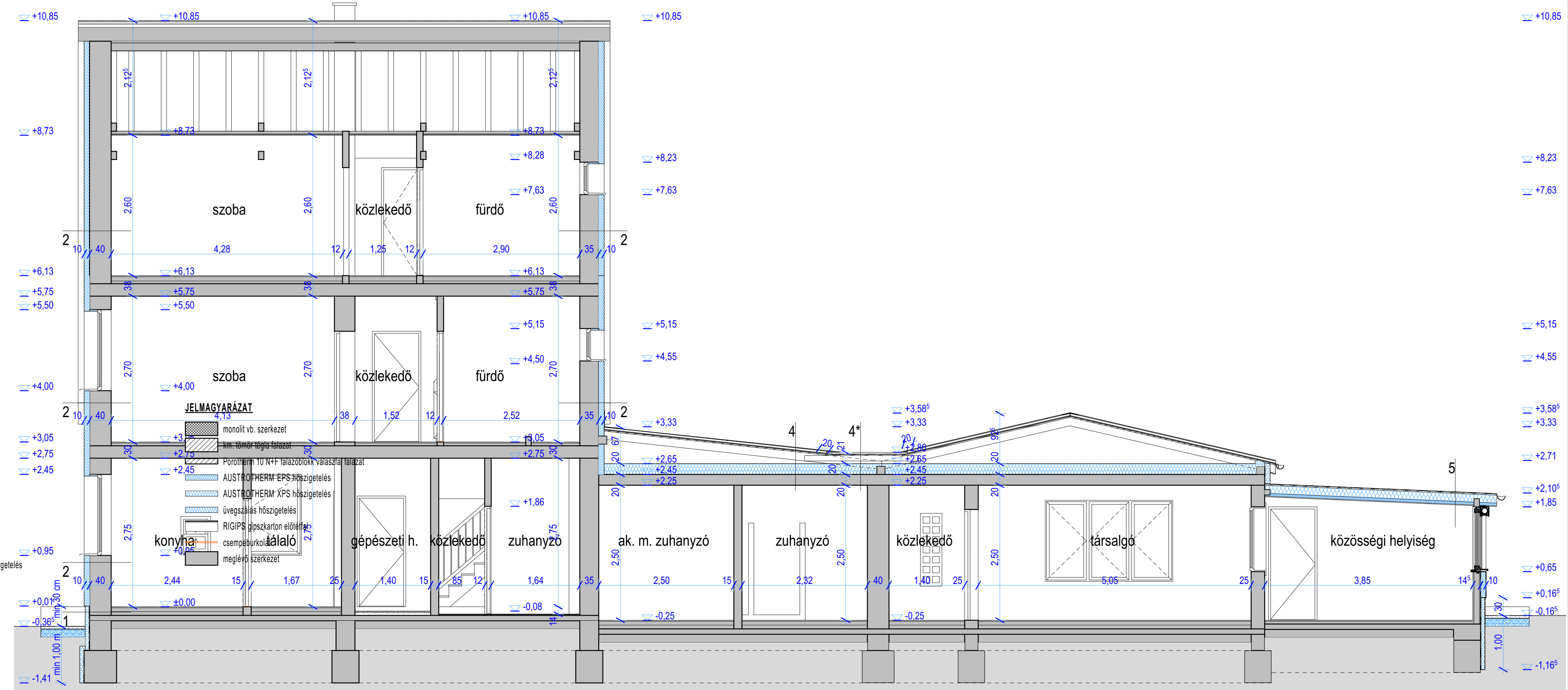
TERVEZETT A-A METSZET m=1:50
