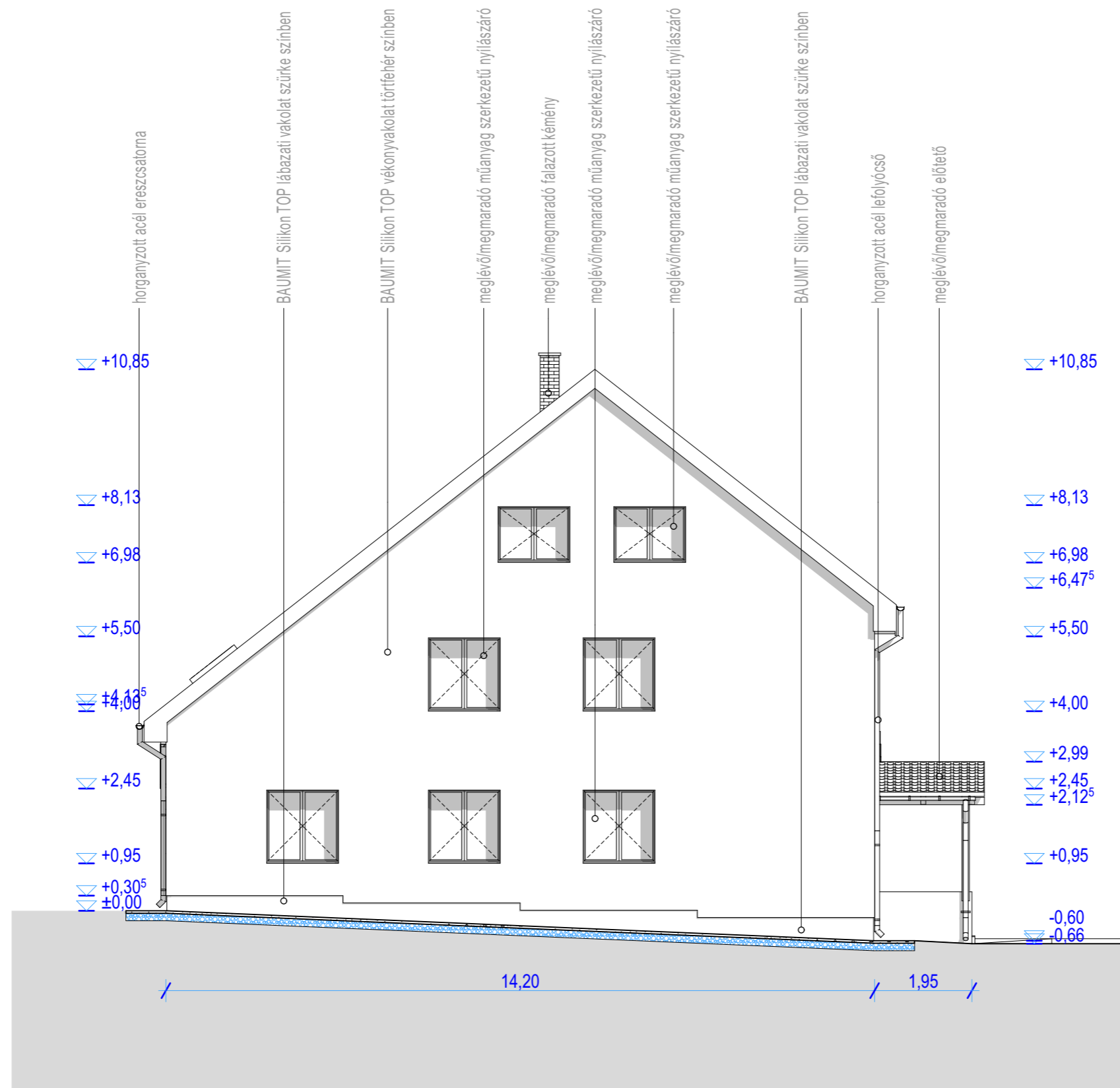
TERVEZETT ÉSZAKI HOMLOKZAT m=1:100
