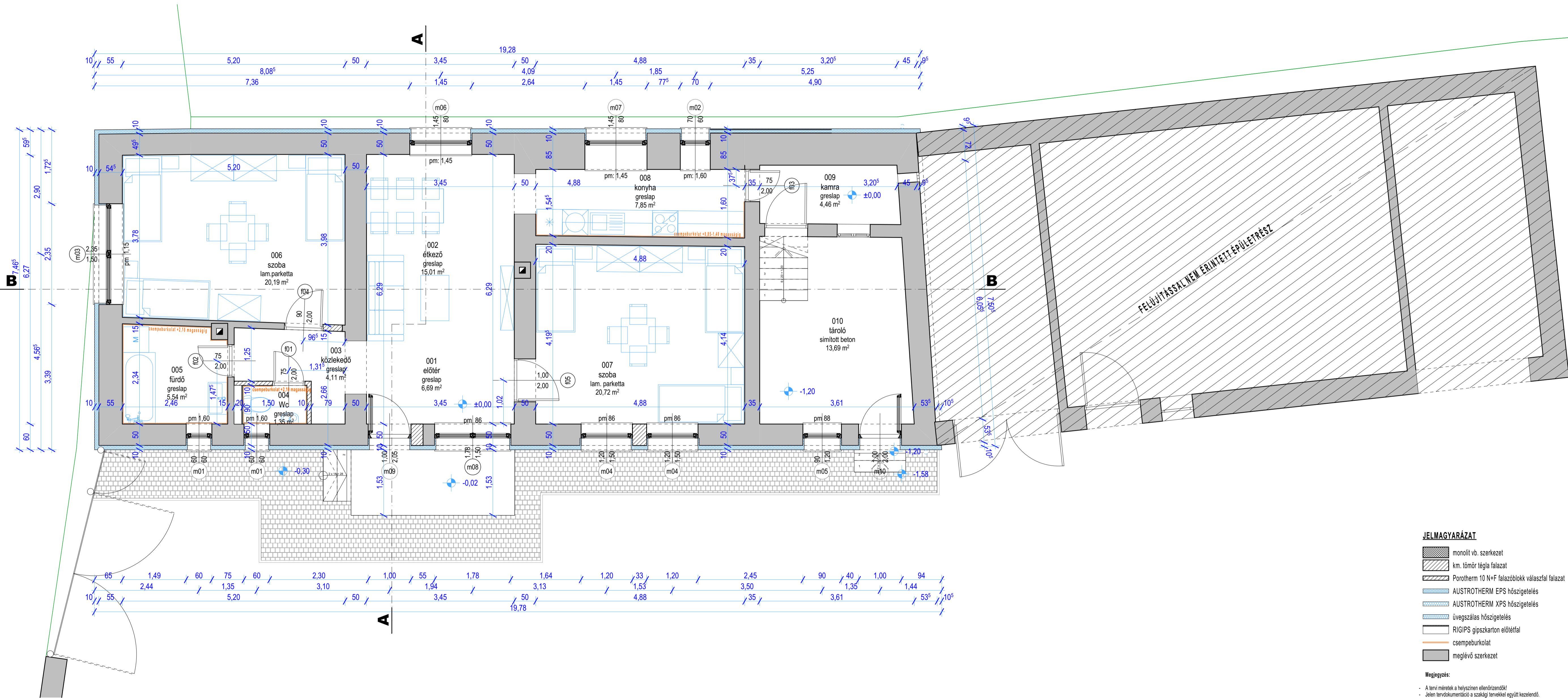
TERVEZETT FÖLDSZINTI ALAPRAJZ m=1:50
