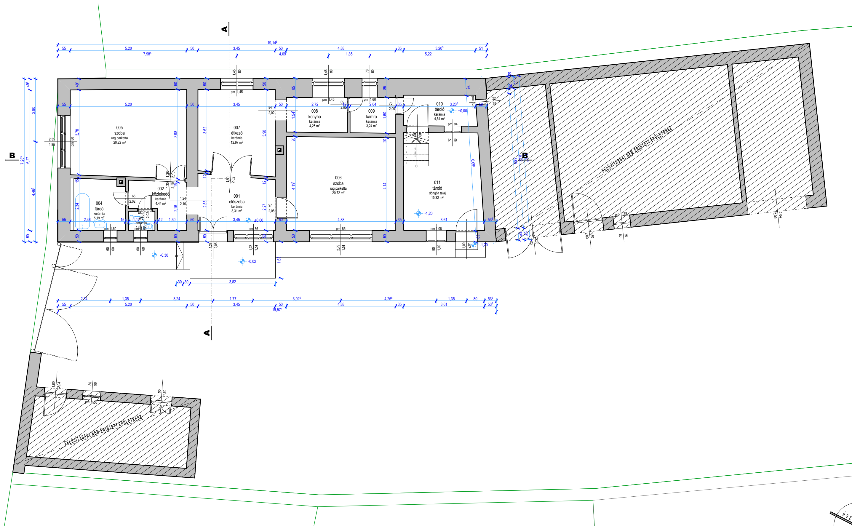
FELMÉRÉSI FÖLDSZINTI ALAPRAJZ m=1:100
